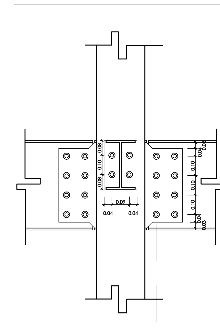
4 12 Detalle de unión 2 Adecuación Mercado Municipal Esc. 1:100
