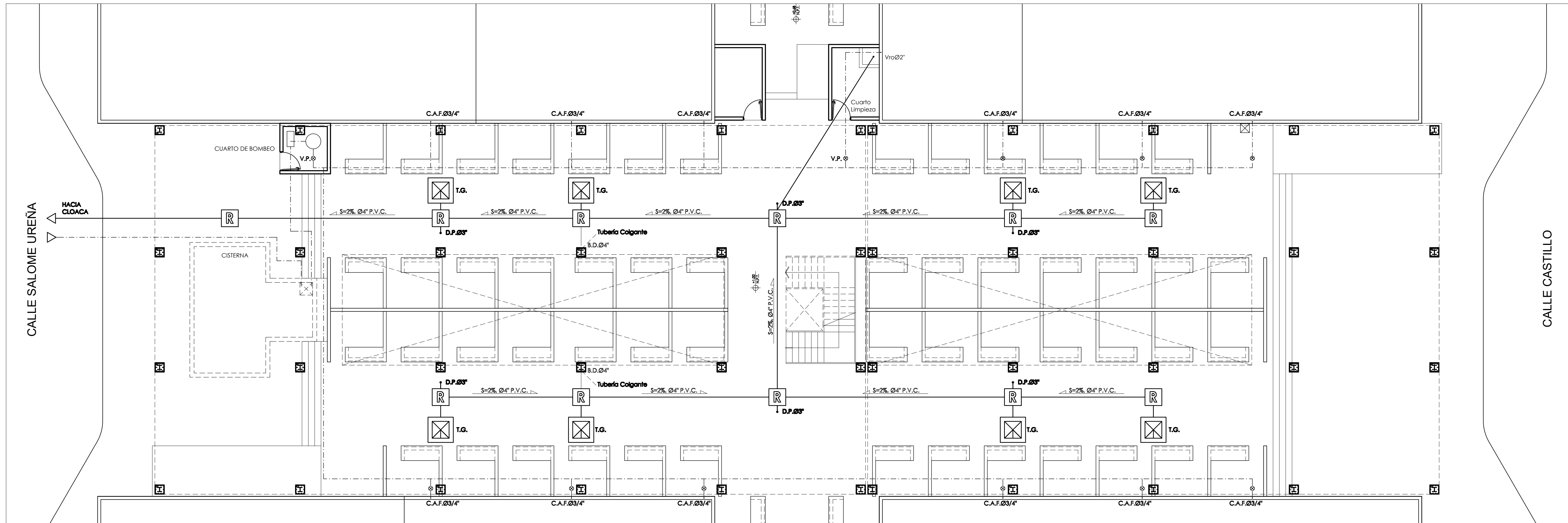
1 14 Instalación de Aguas Residuales y Potable Adecuación Mercado Municipal • 1er. Nivel Esc. 1:100
