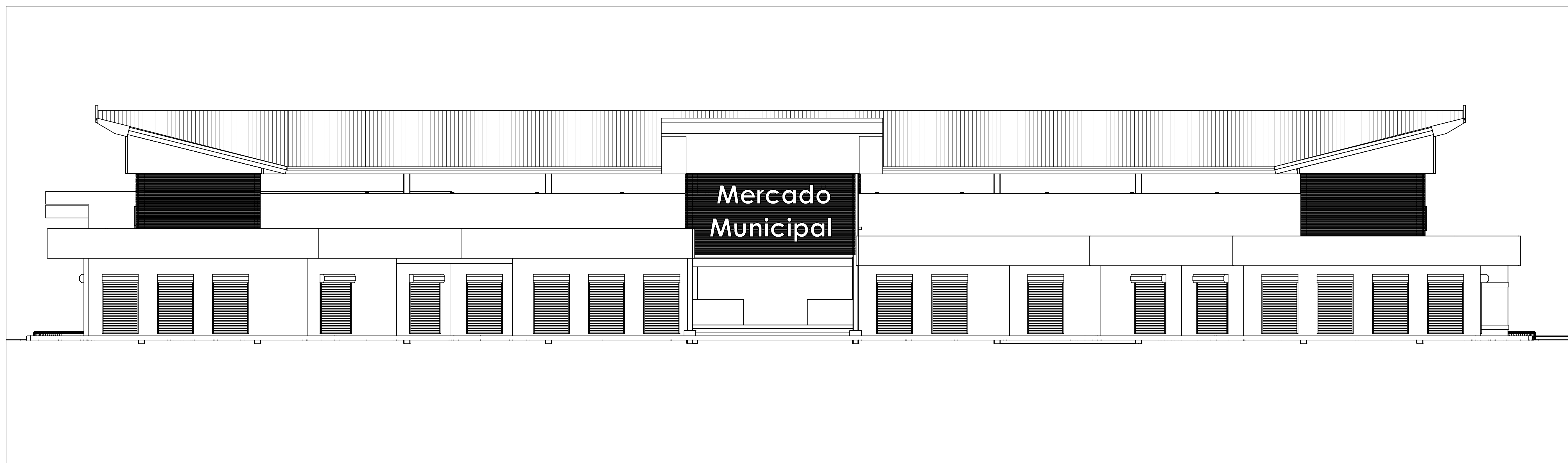
2 7 Elevación Calle Sánchez Adecuación Mercado Municipal Esc. 1:100
