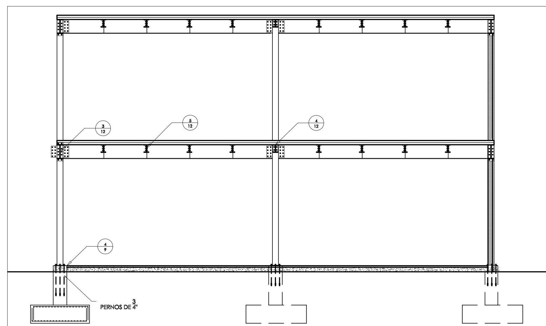
2 12 Detalle de pórtico, Sección B-B Adecuación Mercado Municipal • 2do. Nivel Esc. 1:75
