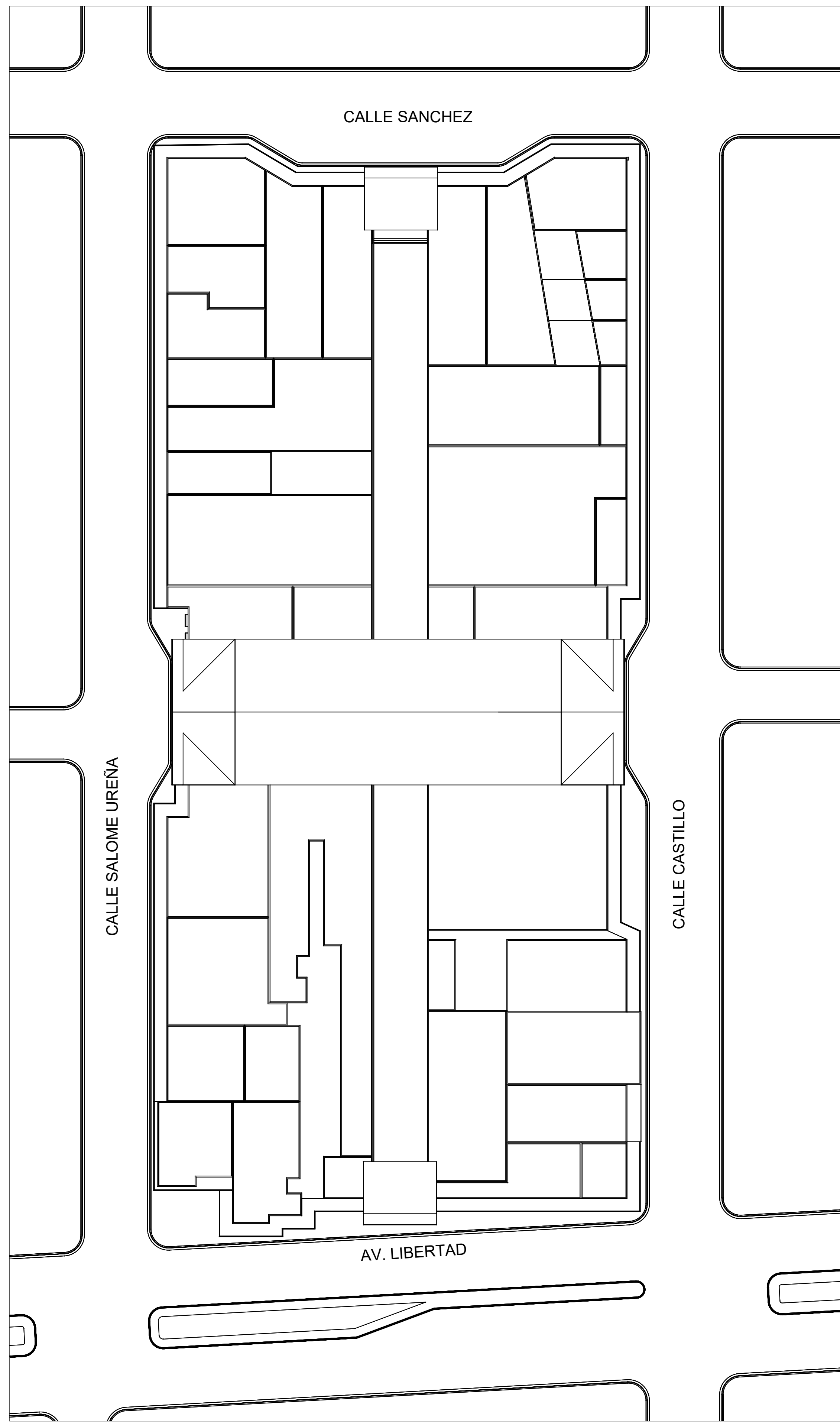
1 Planta Arquitectónica de Conjunto Adecuación Mercado Municipal Esc. 1:400
