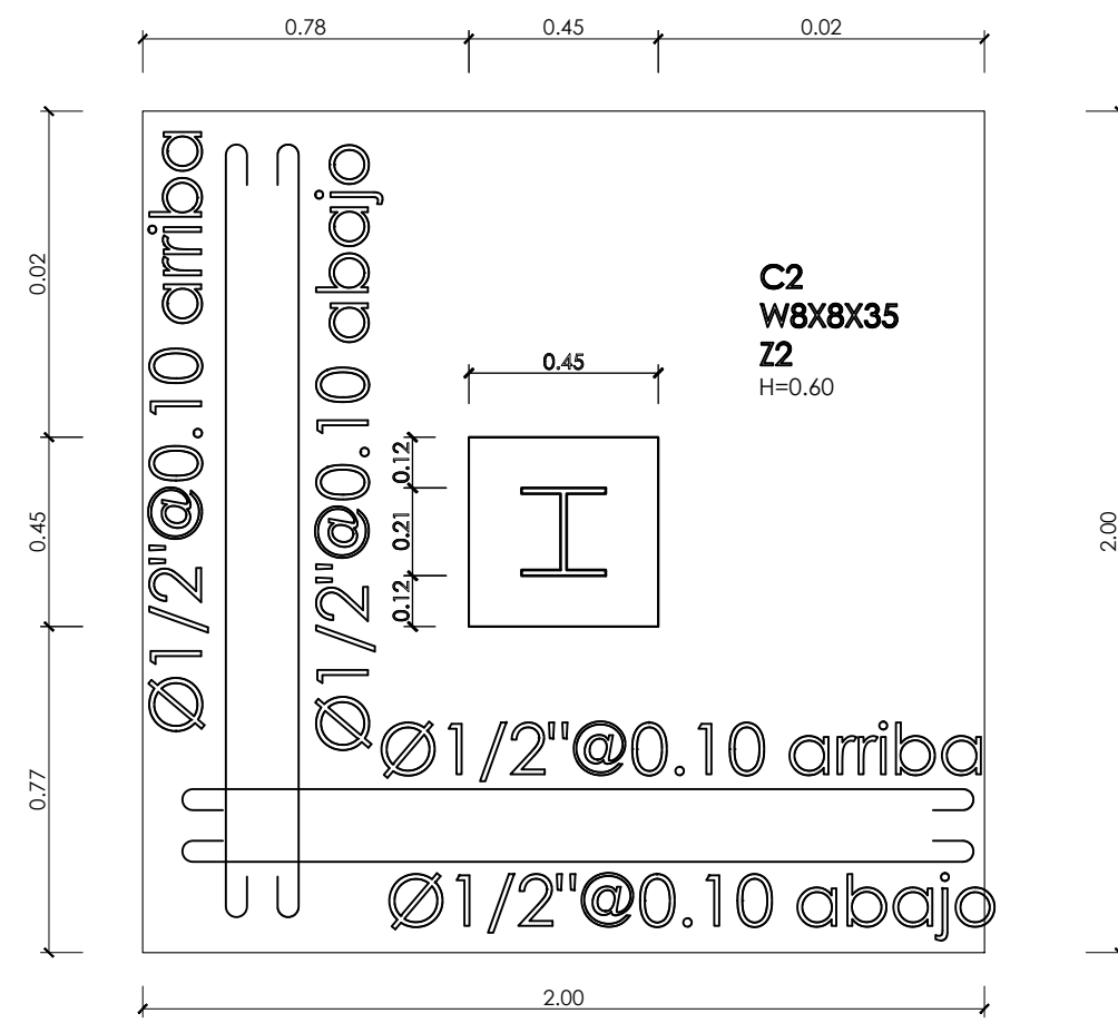
3 9 Detalles de zapatas Adecuación Mercado Municipal Esc. 1:20
