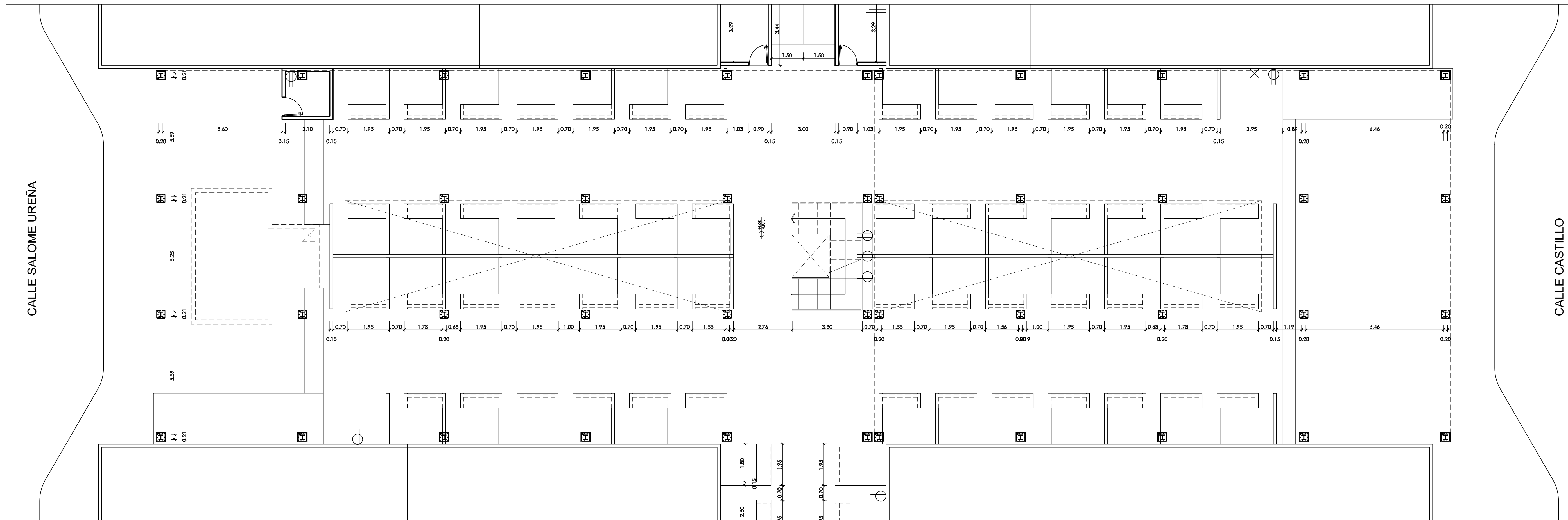
1 6 Planta Dimensionada Módulo B Adecuación Mercado Municipal • 1er. Nivel Esc. 1:100
