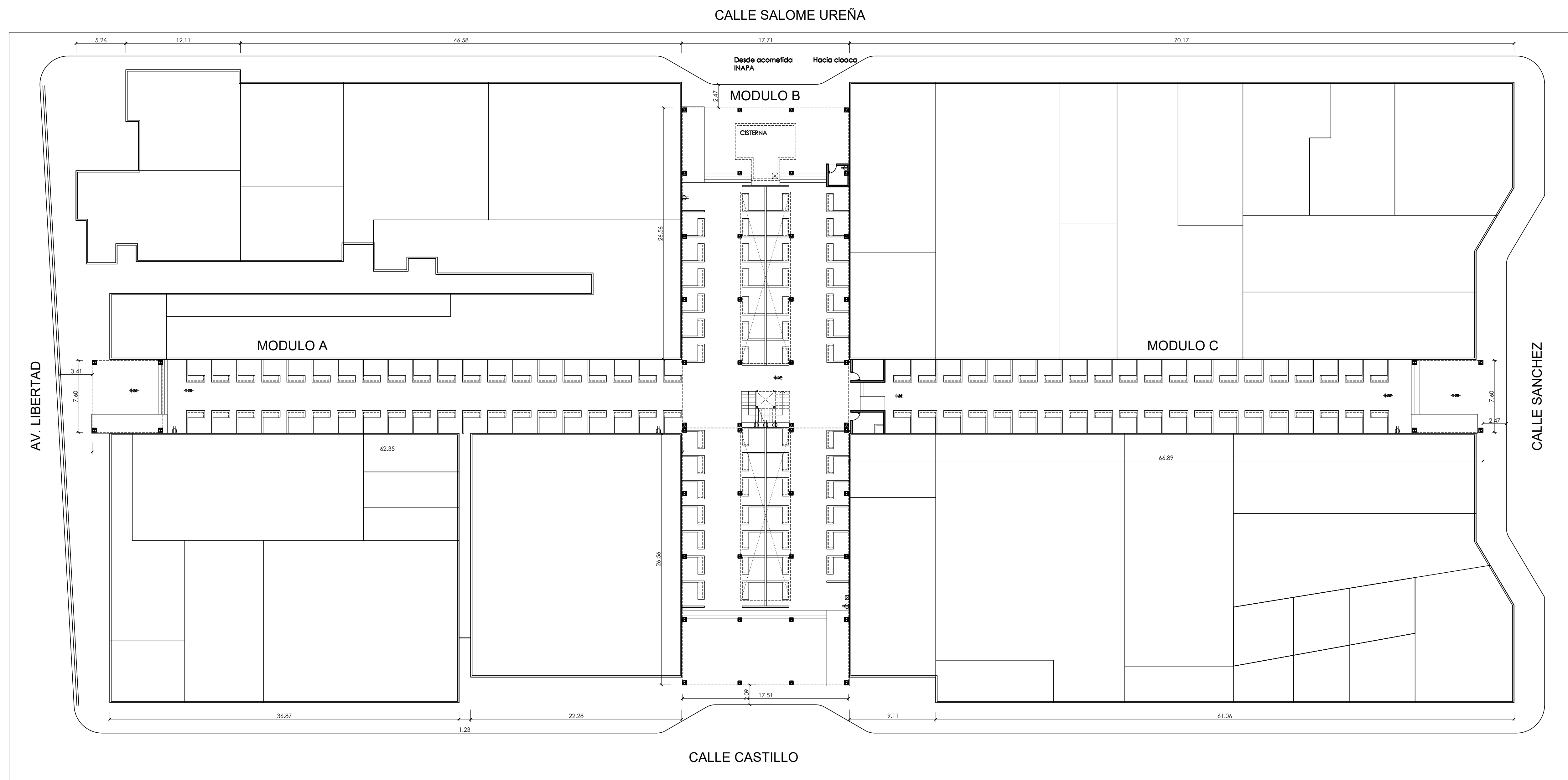
1 2 Planta Arquitectónica de Conjunto Adecuación Mercado Municipal Esc. 1:250
