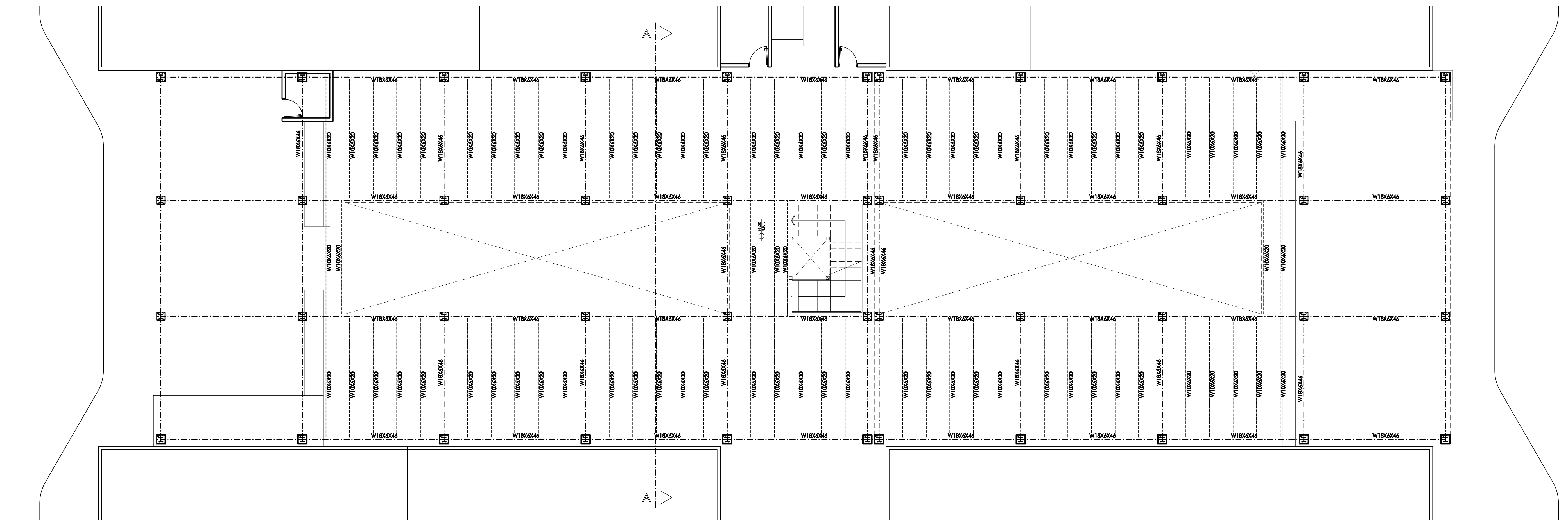
2 11 Planta de Entrepiso Módulo B Adecuación Mercado Municipal • 1er. Nivel Esc. 1:100
