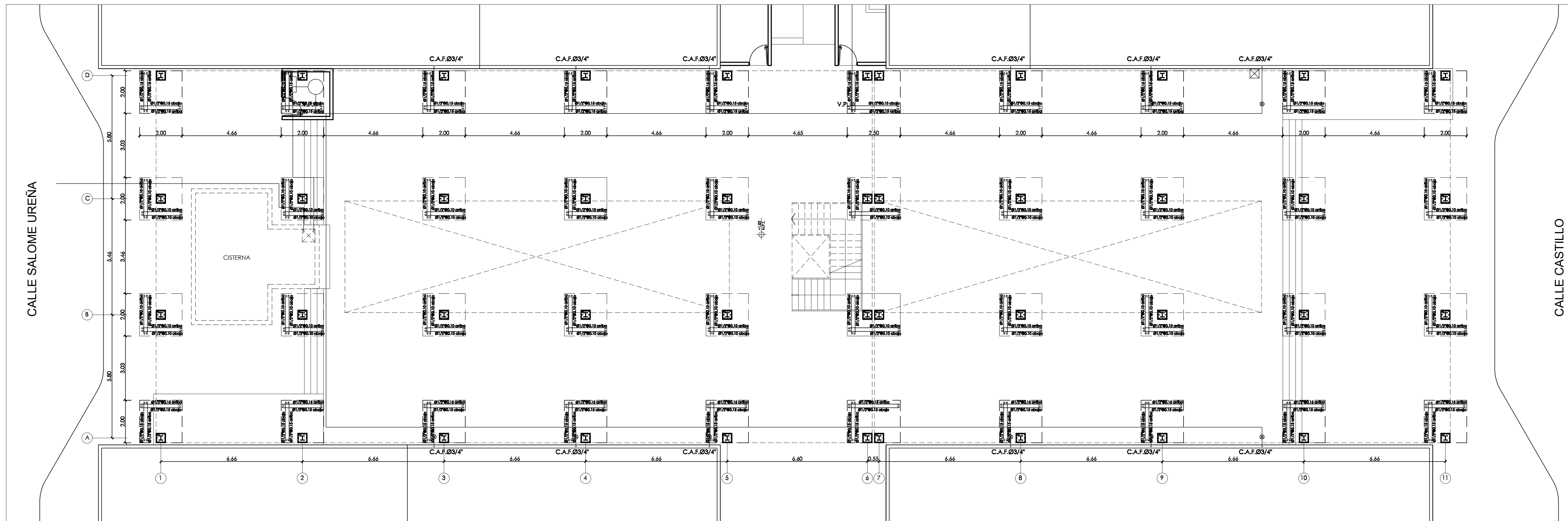
1 11 Planta Cimentaciones Módulo B Adecuación Mercado Municipal • 1er. Nivel Esc. 1:100
