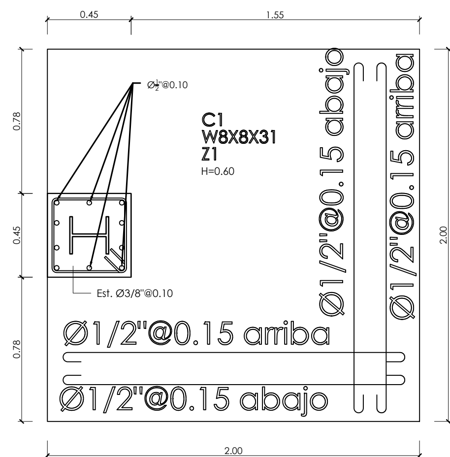
3 9 Detalles de zapatas Adecuación Mercado Municipal Esc. 1:20
