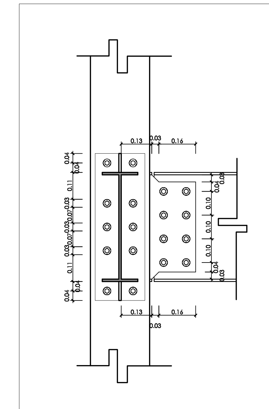
3 12 Detalle de unión 1 Adecuación Mercado Municipal Esc. 1:100
