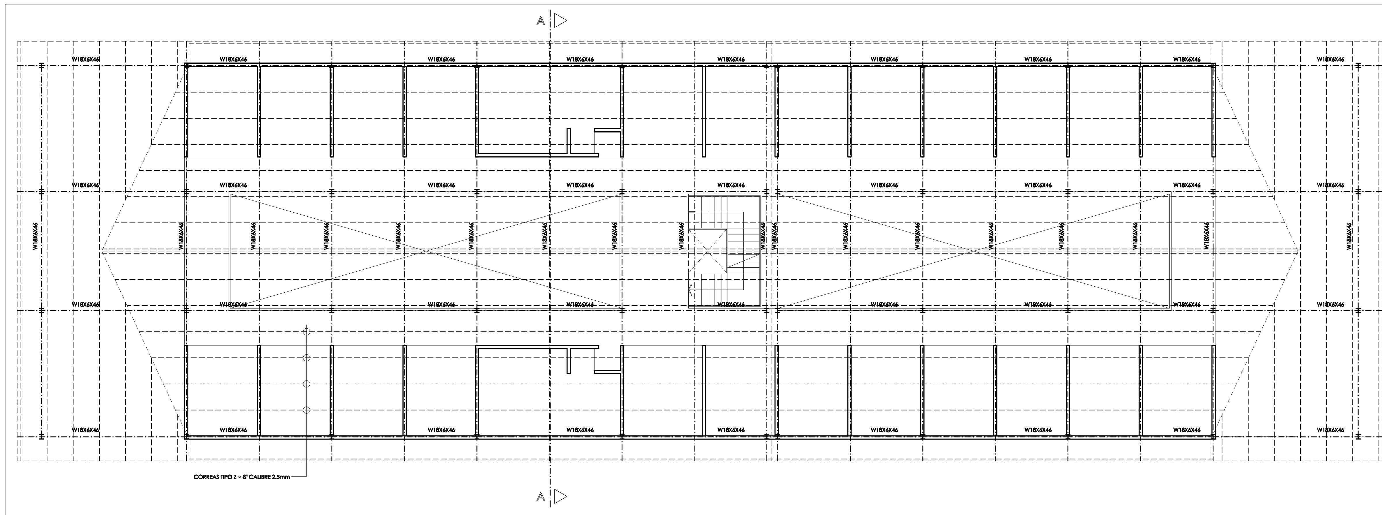
1 12 Planta de Techo Módulo B Adecuación Mercado Municipal • 2do. Nivel Esc. 1:100
