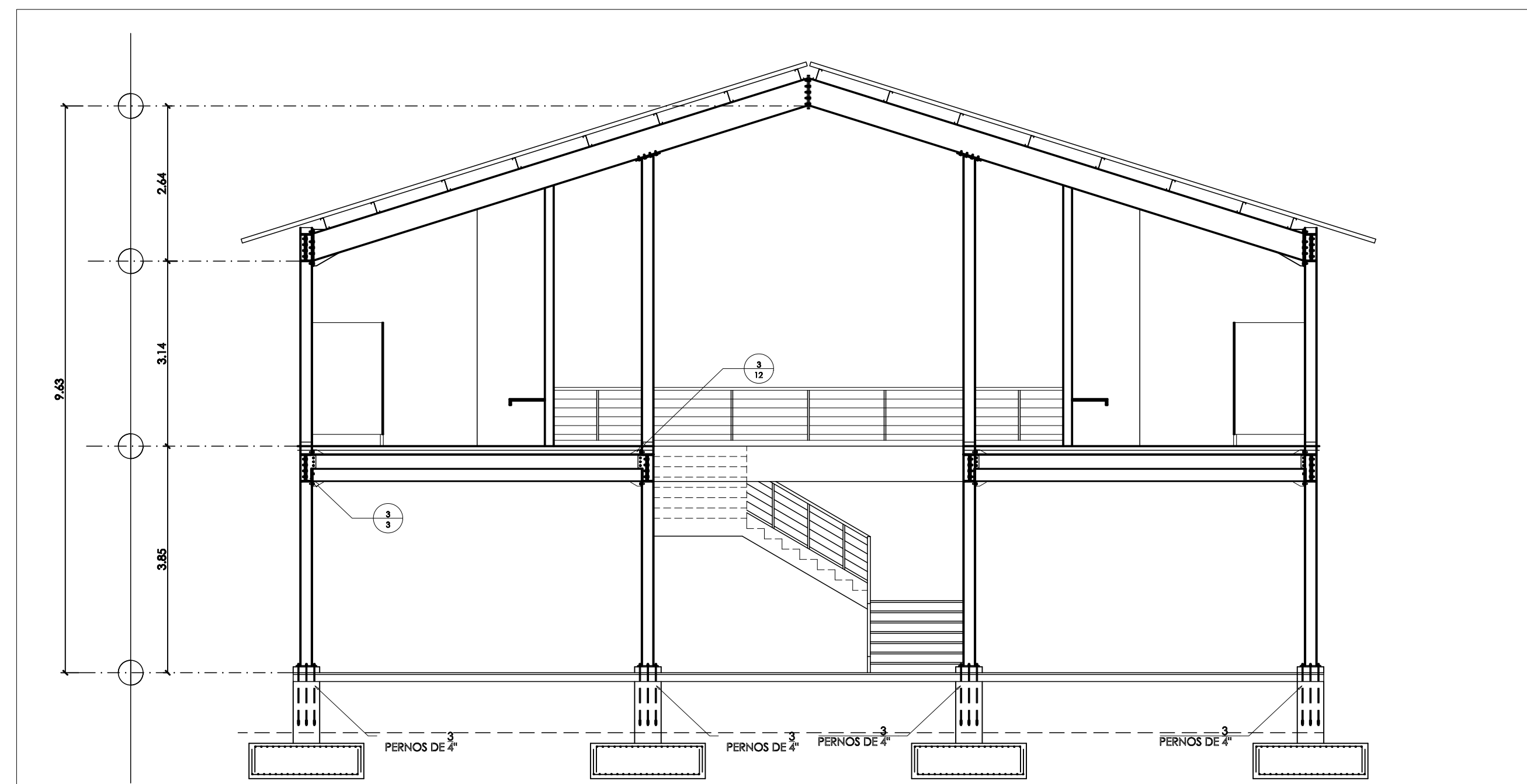
2 12 Detalle de pórtico, Sección A-A Adecuación Mercado Municipal • 2do. Nivel Esc. 1:75
