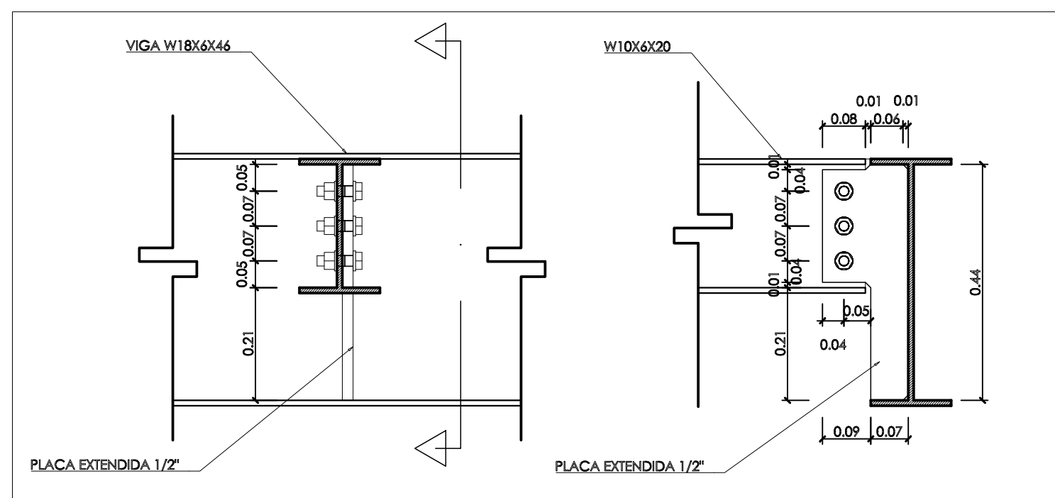
5 12 Detalle de unión 3 Adecuación Mercado Municipal Esc. 1:100
