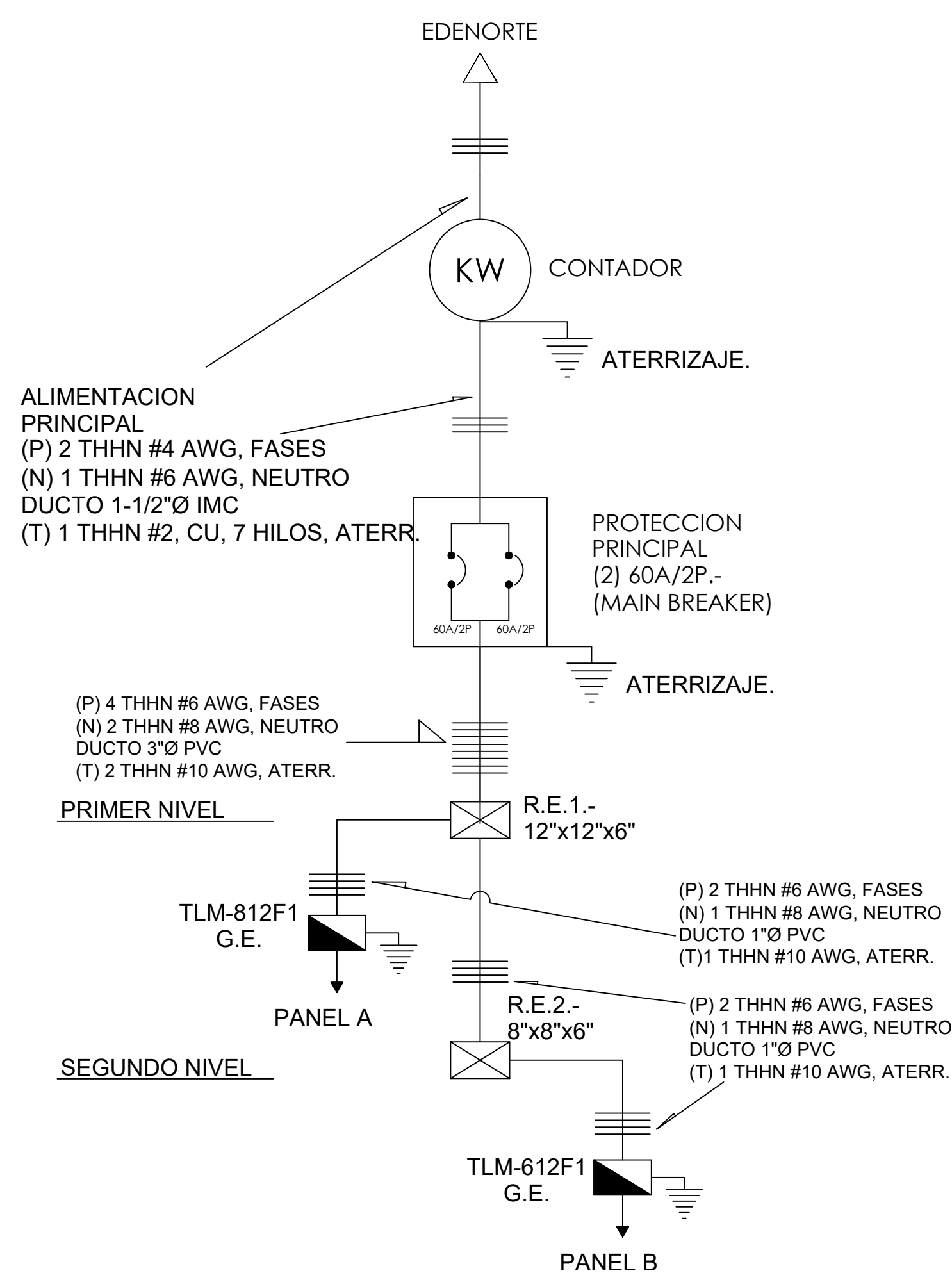
DIAGRAMA UNIFILAR DE POTENCIA
