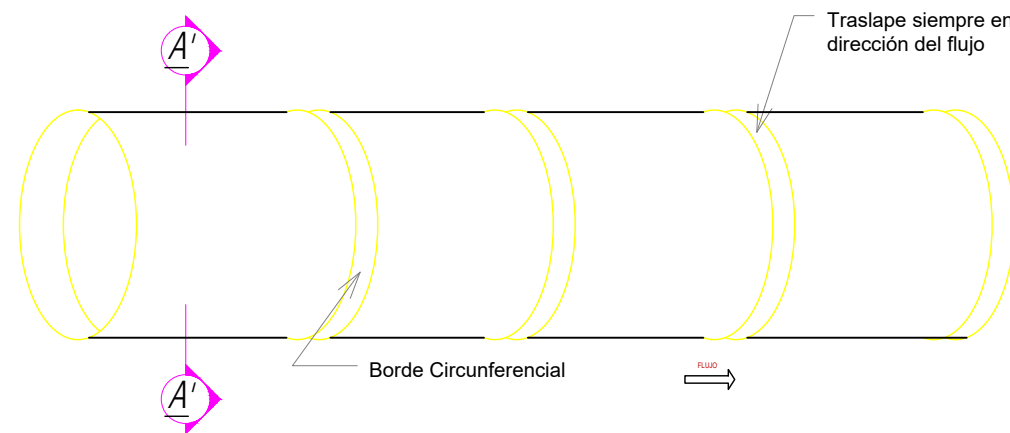
DETALLE ALCANTARILLA EN CONCRETO
