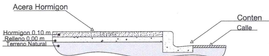
Detalle Acera
