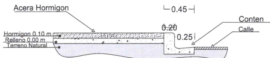
Detalle Acera
