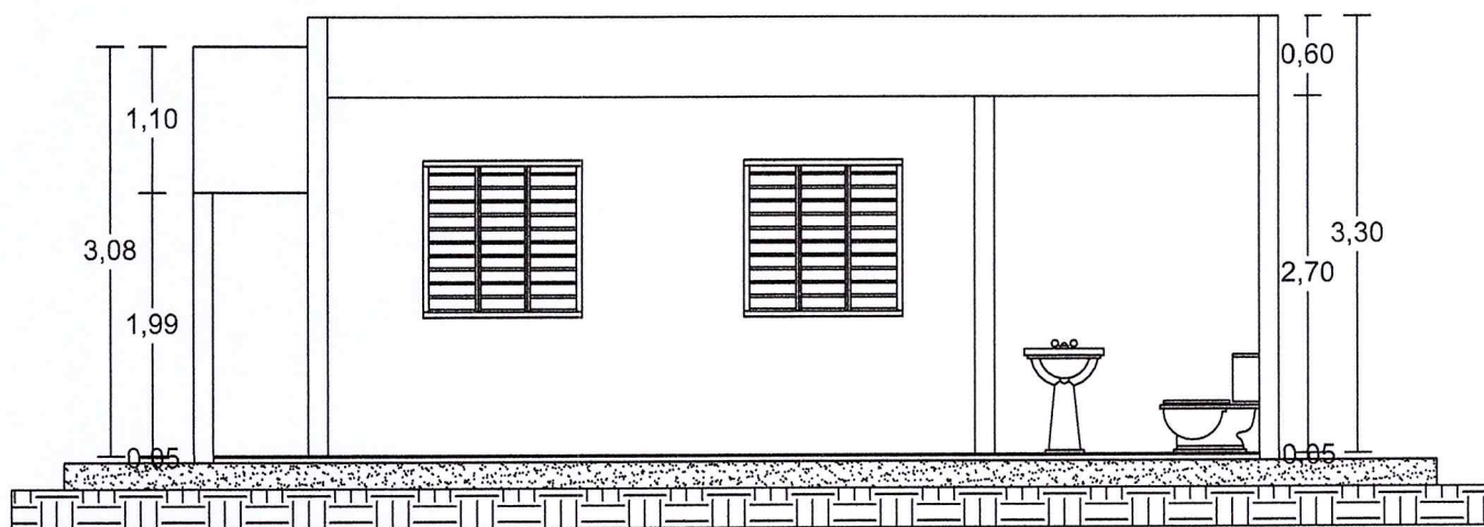
SECCION A-Á
