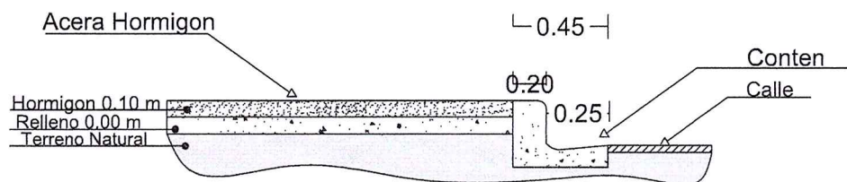
Detalle Acera
