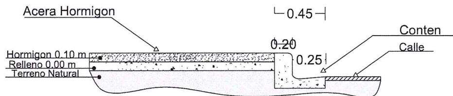
Detalle Acera
