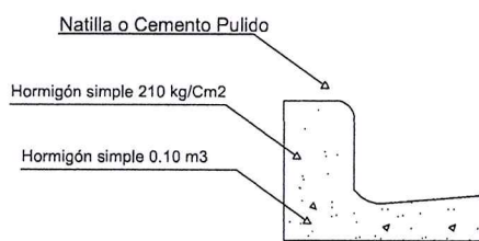
Detalle Acera
