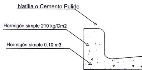
Detalle Terminación Conten
