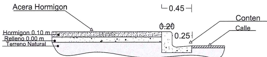
Detalle Acera
