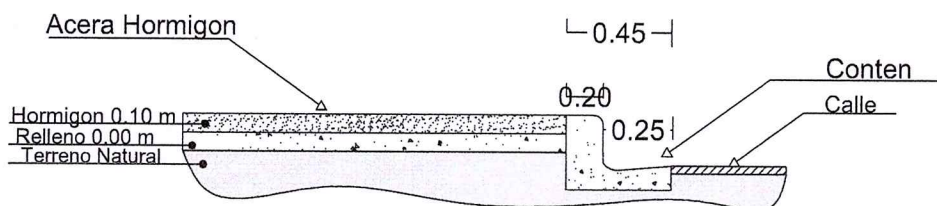
Detalle Acera
