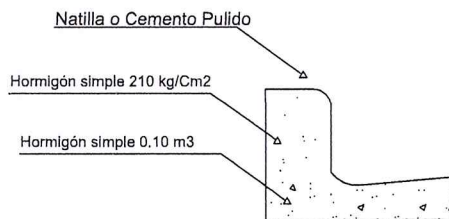
Detalle Terminación Conten
