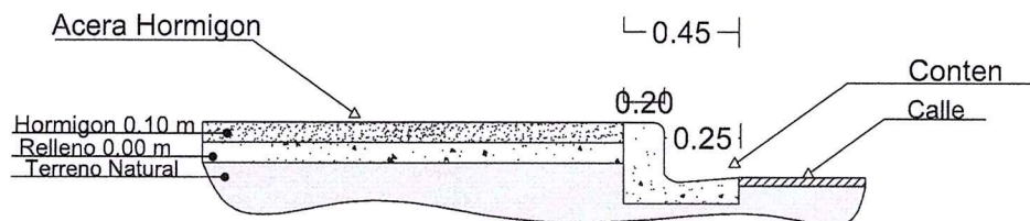
Detalle Acera
