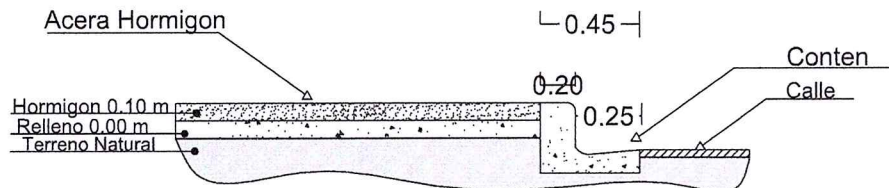
Detalle Acera
