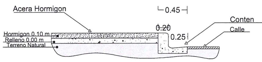
Detalle Acera
