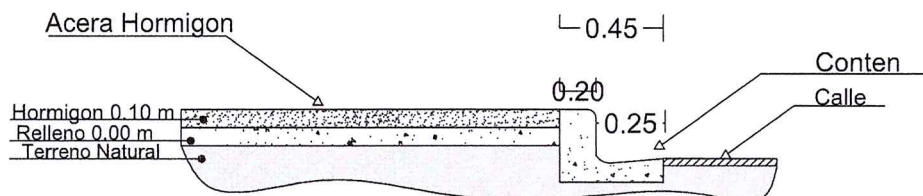
Detalle Acera
