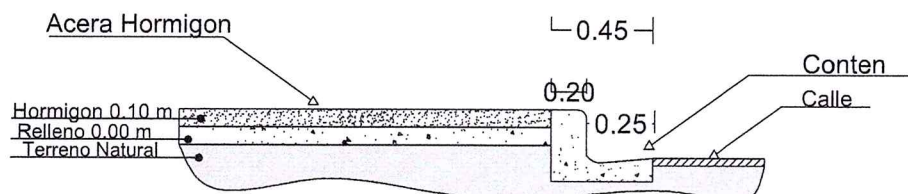
Detalle Acera
