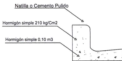
Detalle Terminación Conten
