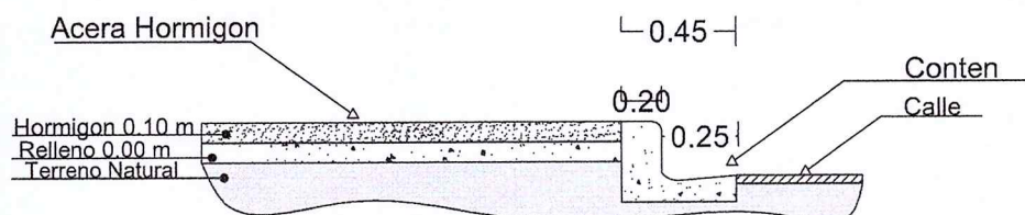
Detalle Acera
