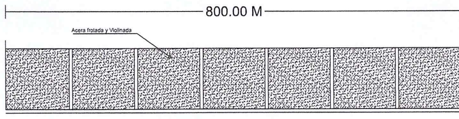
Vista en Planta Acera
