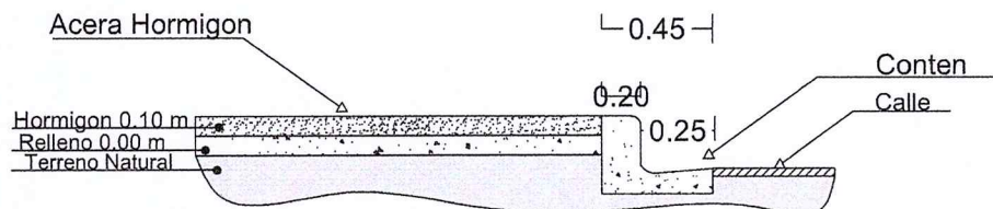
Detalle Acera
