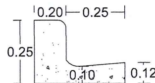
Detalle Contén
