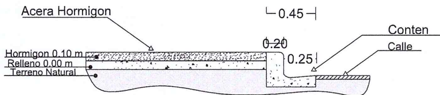
Detalle Acera
