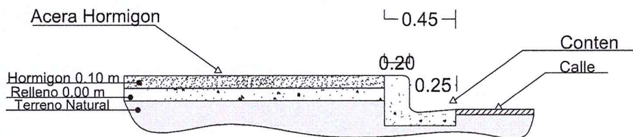
Detalle Acera
