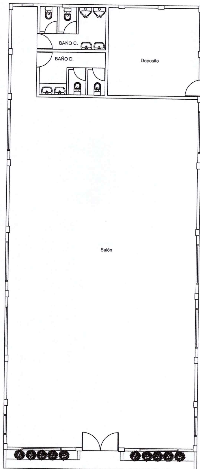
PLANTA ARQUITECTONICA AMUEBLADA
