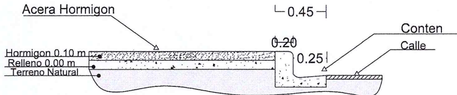
Detalle Acera
