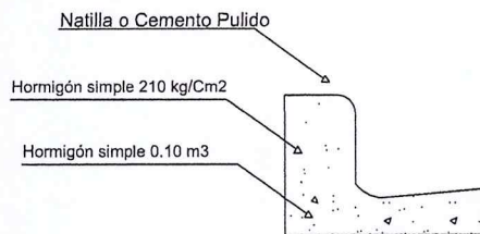
Detalle Terminación Contén
