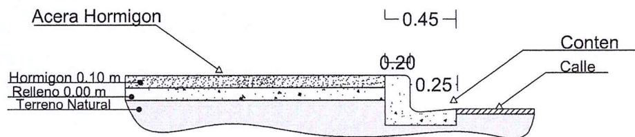
Detalle Acera
