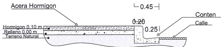
Detalle Acera
