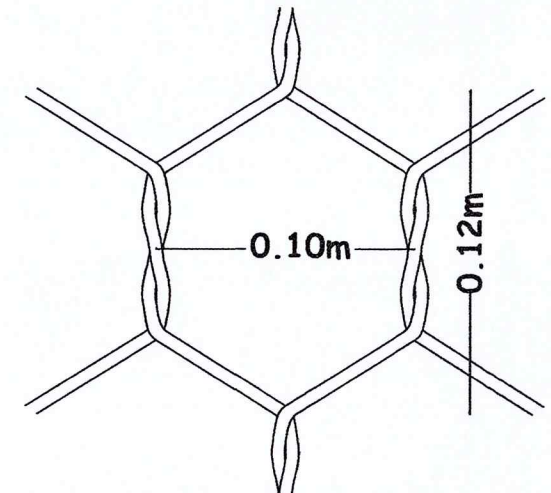
Detalle Malla para muro en gavión
