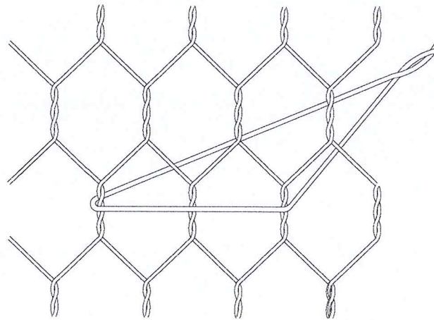
Detalle del Tensor
