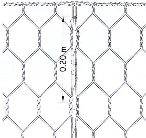
Detalle de la Costura
