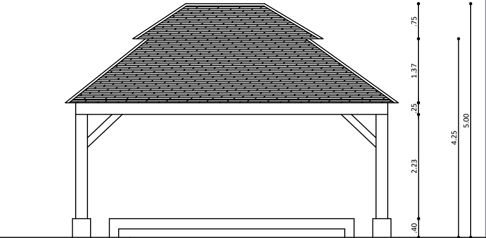
ELEVACION FRONTAL
