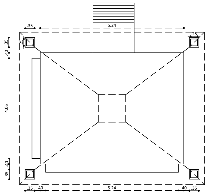
PLANTA ARQUITECTONICA DIMENSIONADA
