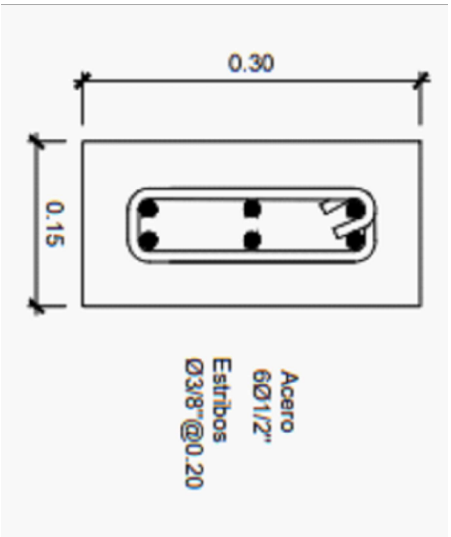
Detalle Detalle ColumnaCG1
