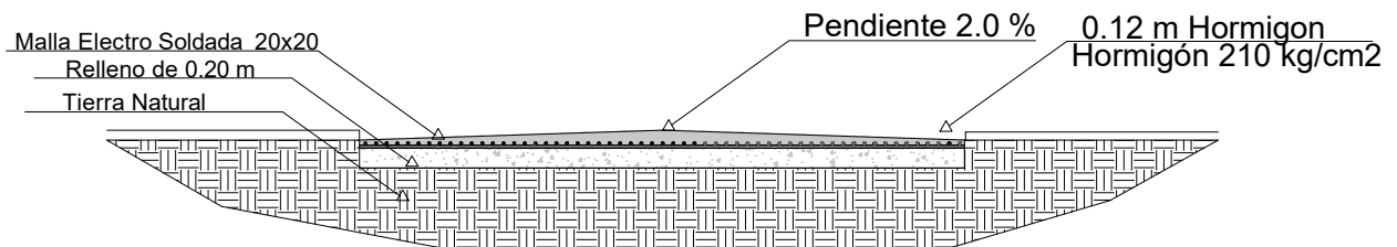
Corte A
