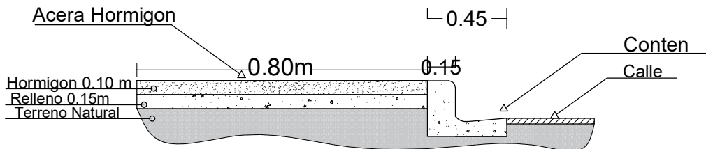
Detalle Acera
