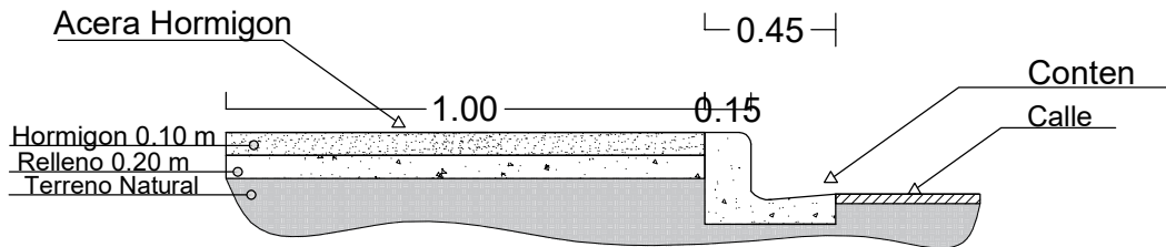
Detalle Acera
