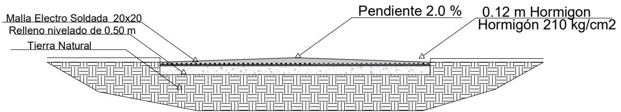
Corte A
