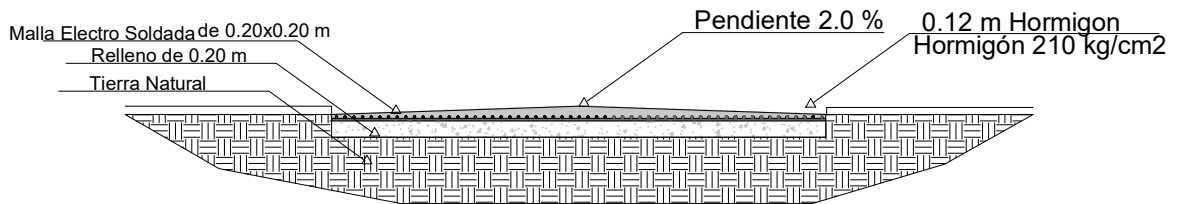
Corte A
