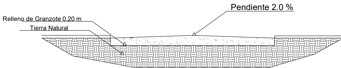
Corte A
