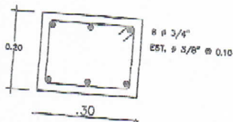
SECCION 3-3' : seccion transversal viga
