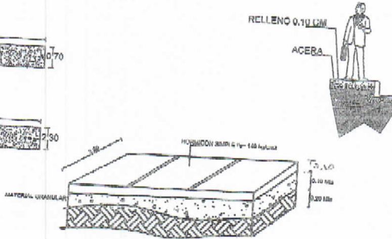
DETALLE ACERAS NO ESC.
