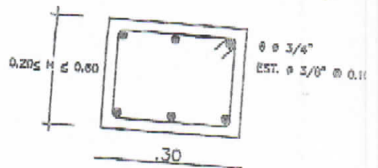
SECCION 2-2' : seccion transversal viga
