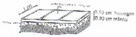
DETALLE ACERAS NO ESC.
