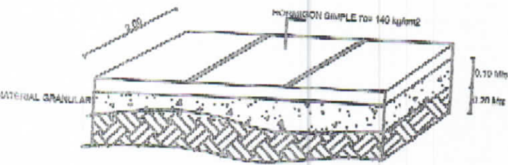
DETALLE ACERAS NO ESC.
