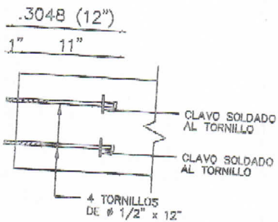
SECCION
