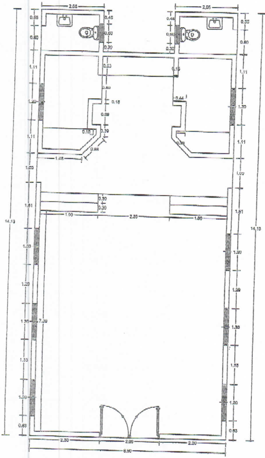
PLANTA DIMENSIONADA CAPILLA
