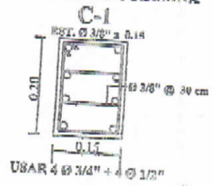
DETALLE DE COLUMNA
