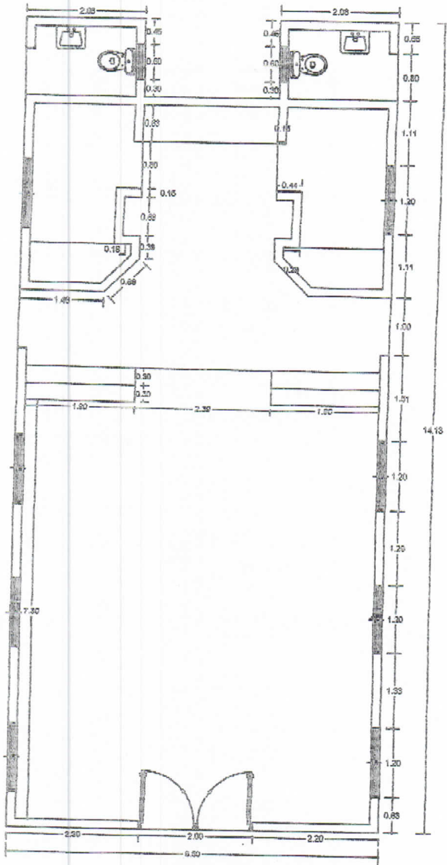
PLANTA DIMENSIONADA
