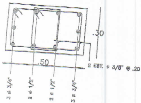
SECCION 1-1' : seccion transversal columna
